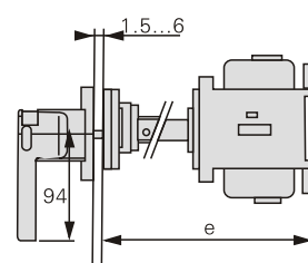
加长轴
