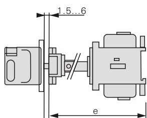
加长轴
