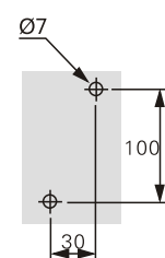
距离 (e) 柜体后部 / 门
